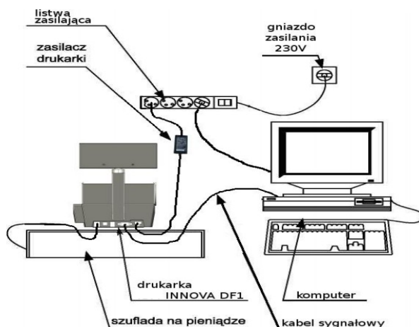
Rysunek 1. Sposób podłączenia drukarki do komputera
